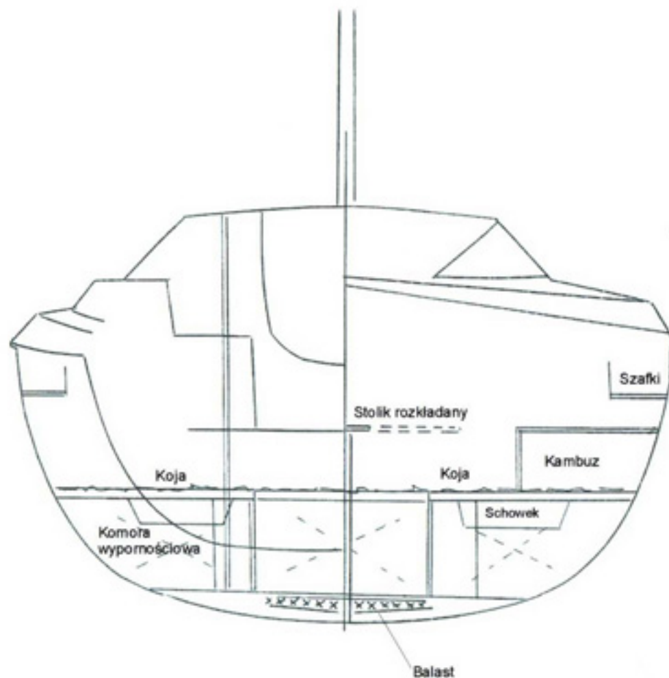
PRZEKRÓJ LEWA BURTA 1:20
